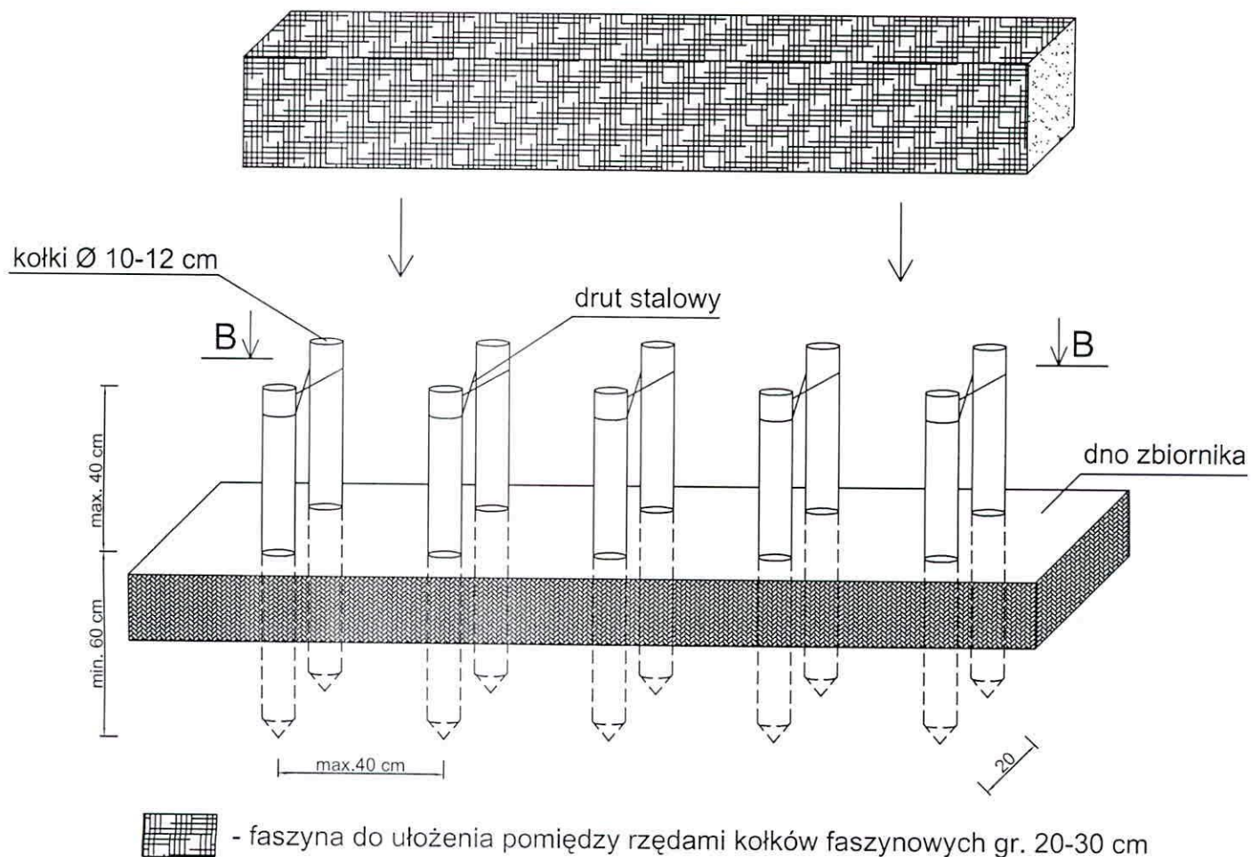
Widok B-B
